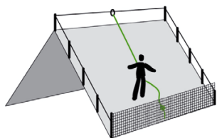
Système de retenue pour toiture de forte pente
