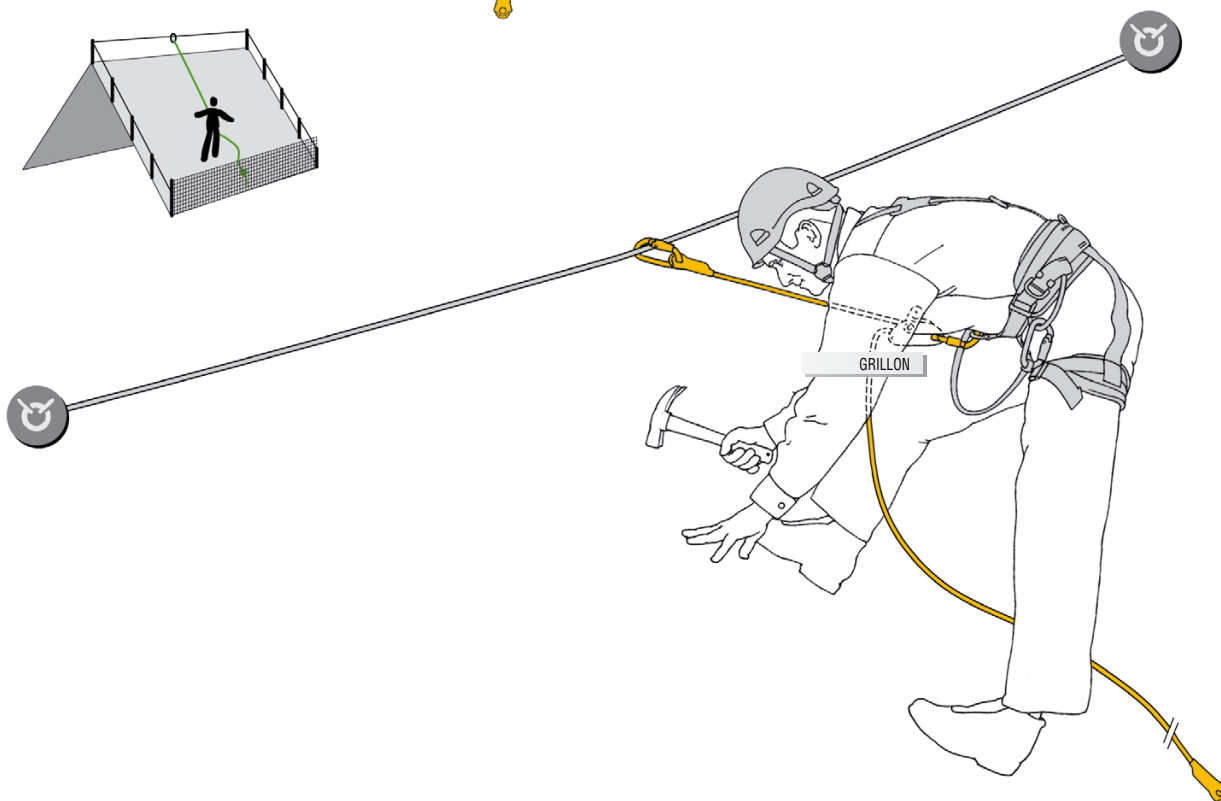
Système de retenue pour toiture de forte pente
